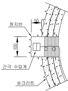
간극수압계
