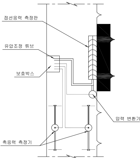
쏜크리트 응력 측정
