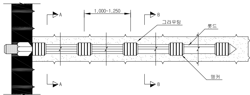
록볼트 축력 측정
