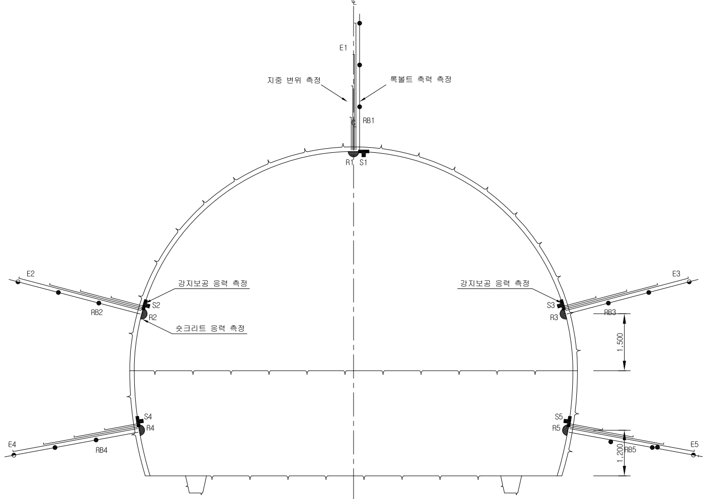
쏜크리트 응력 측정
